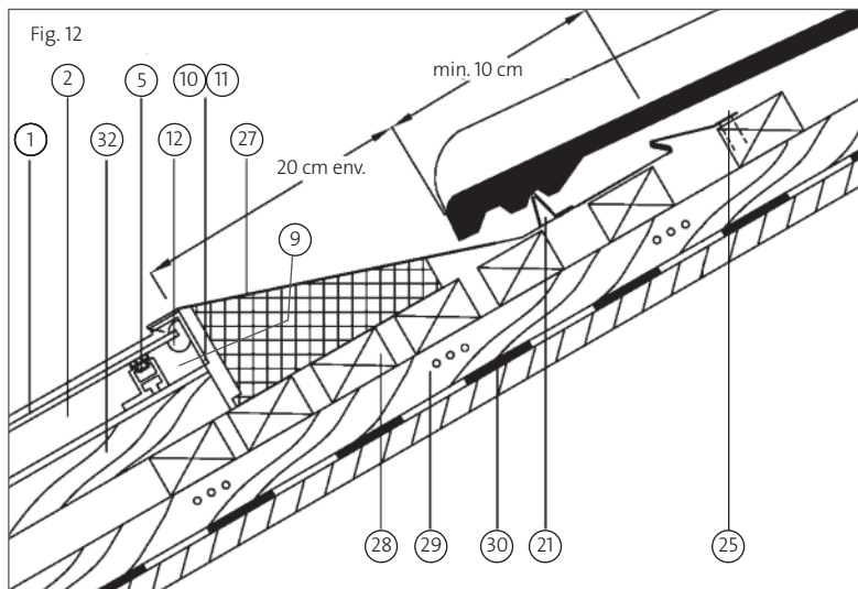
Détail A
