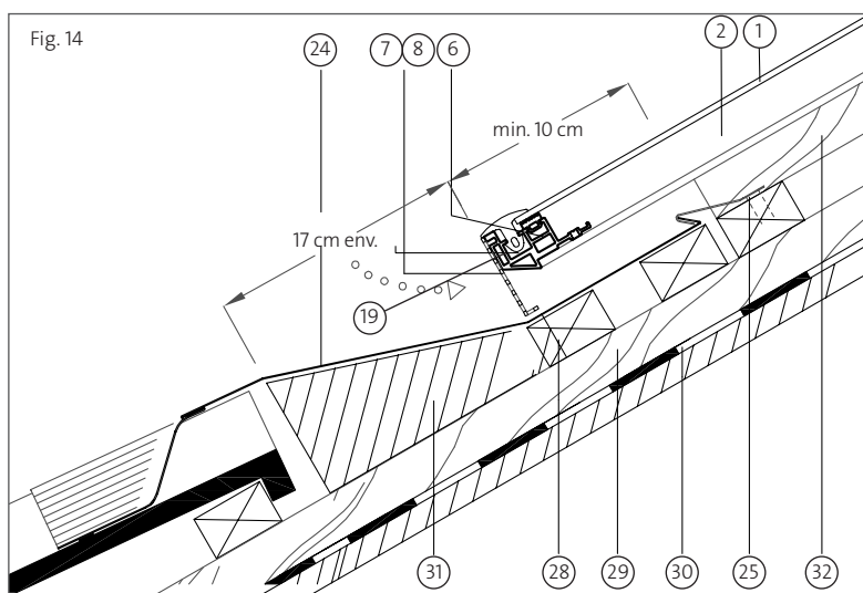
Détail C
