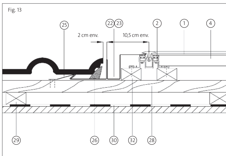
Détail B
